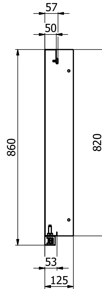
A-A ( 1:10 )
